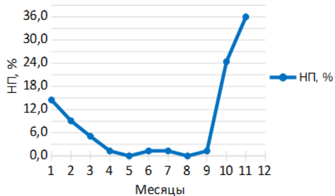
Рис. 22 — Годовой ход СИ и НП
