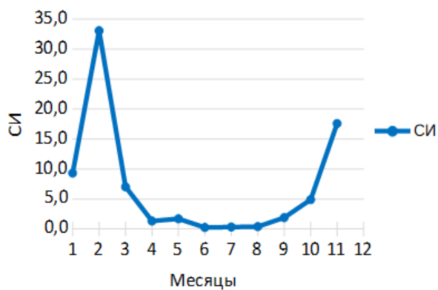
Рис. 4 — Годовой ход СИ и НП
