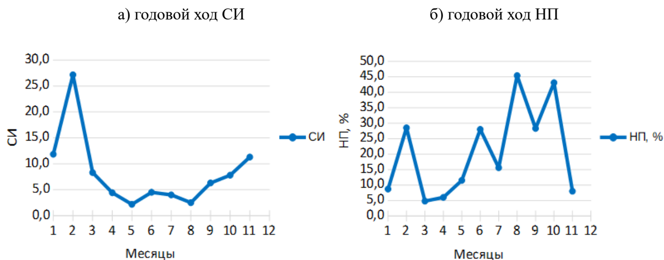
Рис. 6 — Годовой ход СИ и НП
