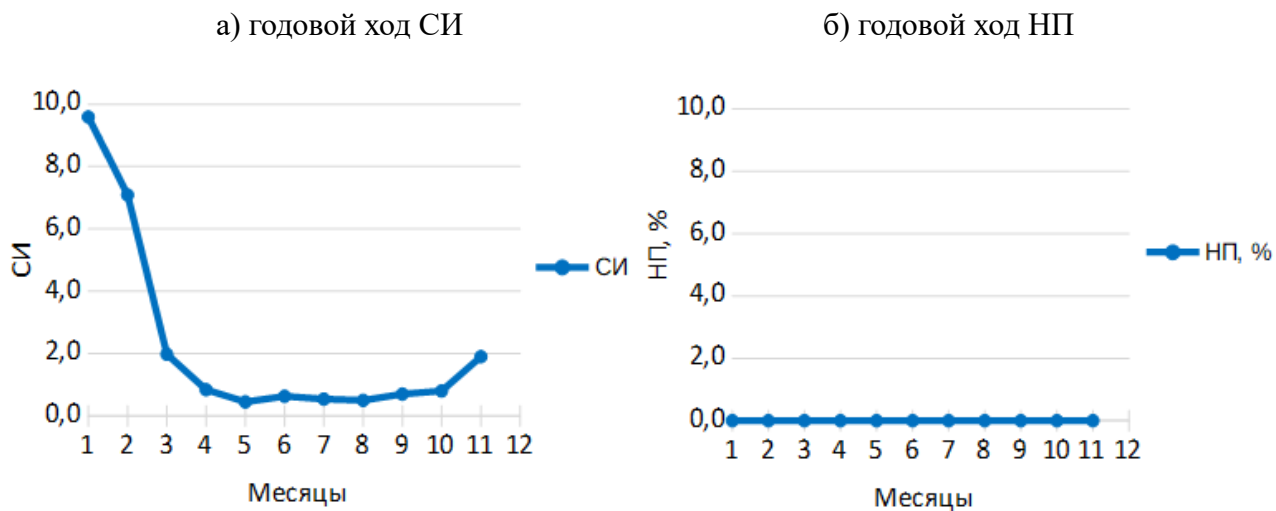
Рис. 20 — Годовой ход СИ и НП
