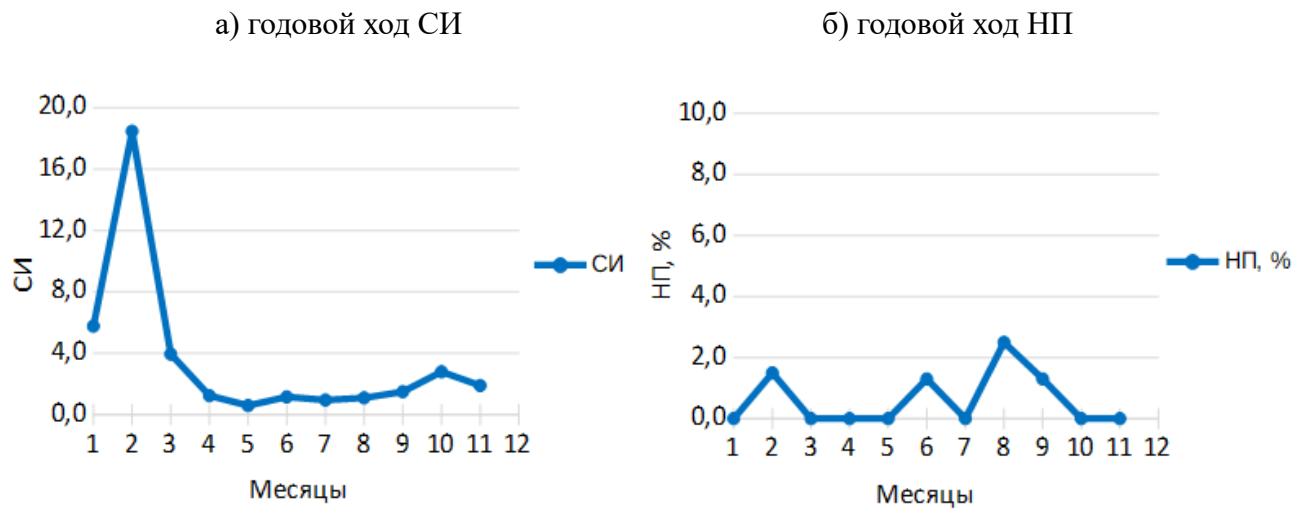
Рис. 12 — Годовой ход СИ и НП
