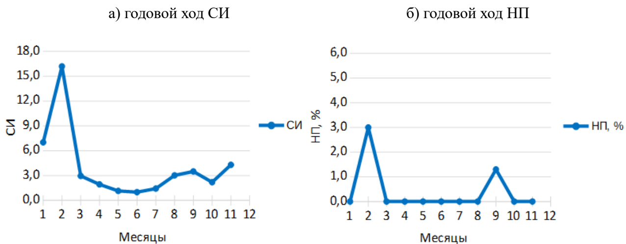
Рис. 8 — Годовой ход СИ и НП
