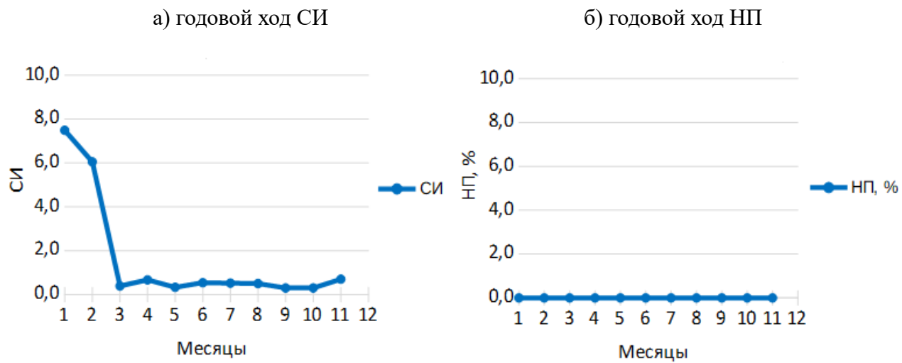
Рис. 18 — Годовой ход СИ и НП
